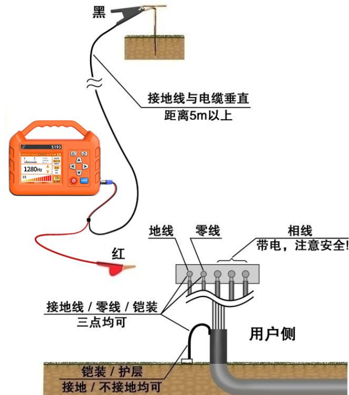
图 27 运行电缆零线 / 地线 / 护层注入法
