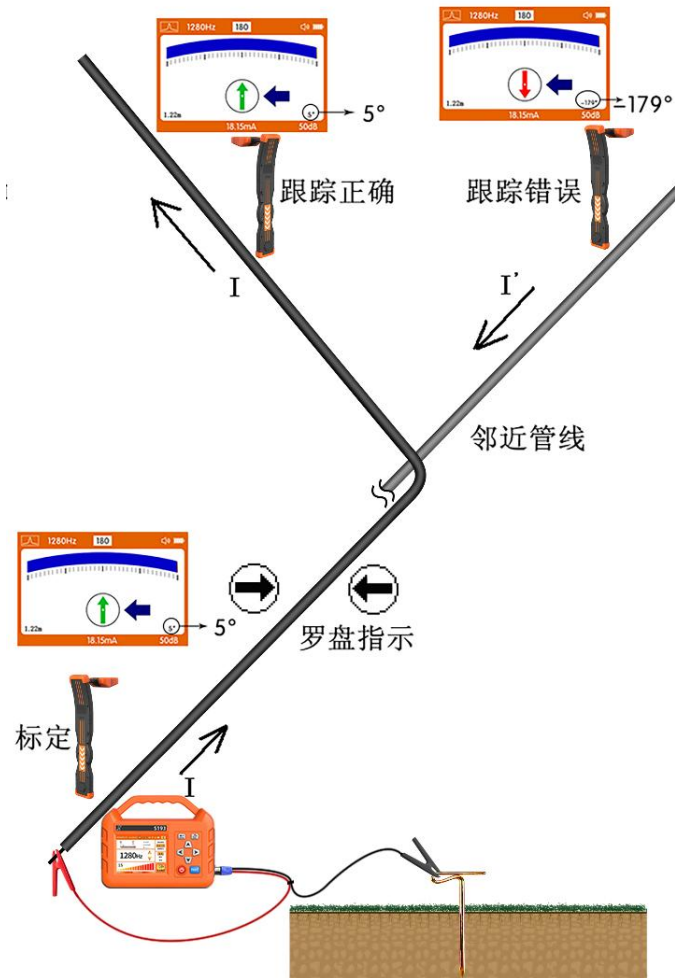
图 34 信号方向跟踪探测过程
