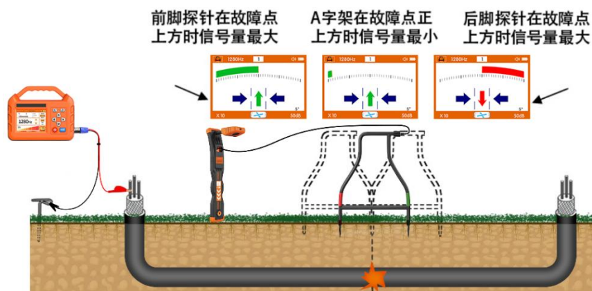
图 66 查障定点
