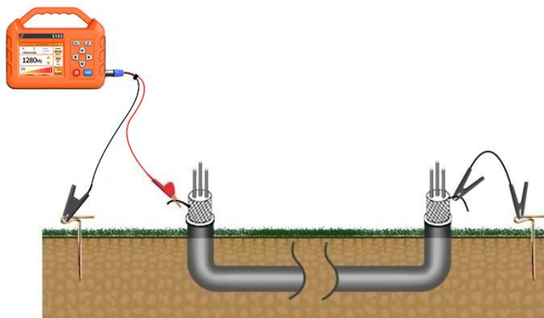
图 64 故障定位发射机接线
