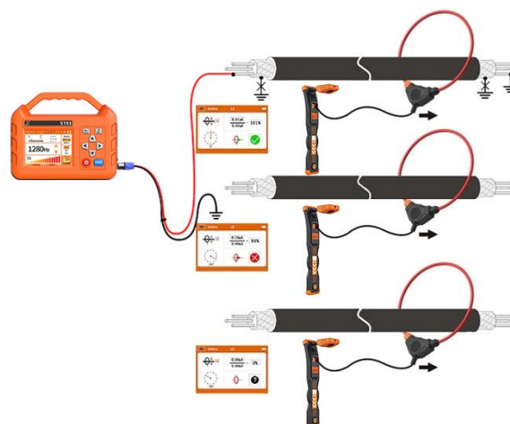
图 45 停电识别(直连法)接线检测
