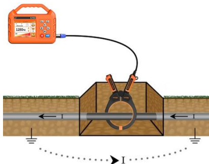
图 21 卡钳耦合接线图
