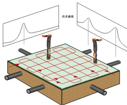
图 36 无源法区域探查
