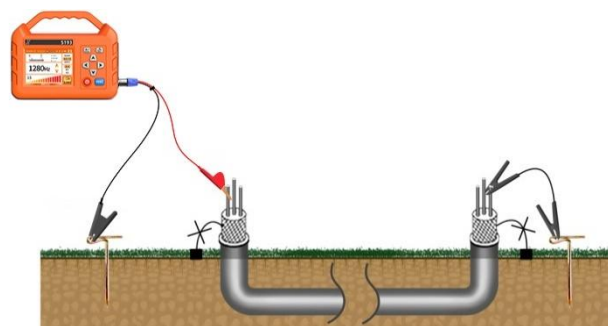
图 10 芯线-大地接法接线图
