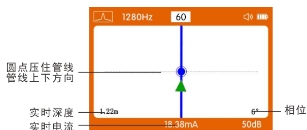
图 40 实时深度和电流测量
