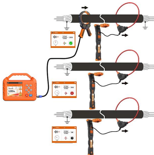
图 46 带电识别(耦合法)接线检测
