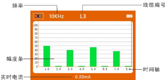
图 49 8.19kHz 以上的电缆识别界面
