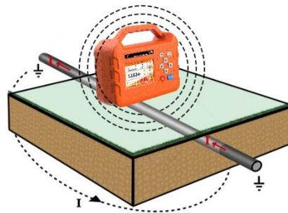
图 26 感应法
