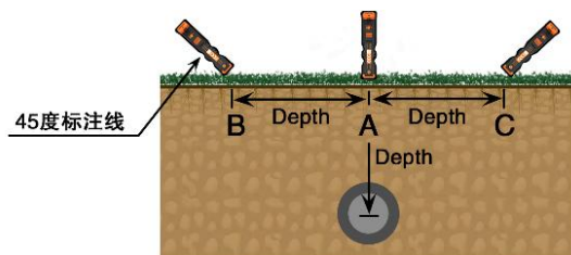
图 41 音谷 45° 法测深
