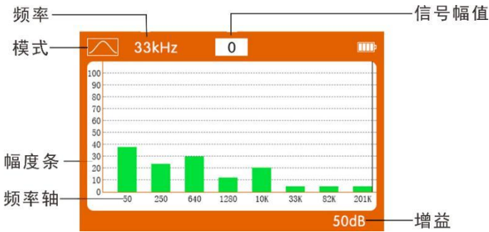
图 69 扫频测试界面
