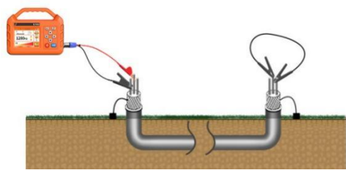
图 17 相间接法接线图
