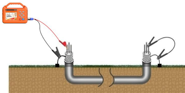
图 14 相线-护层接法接线图
