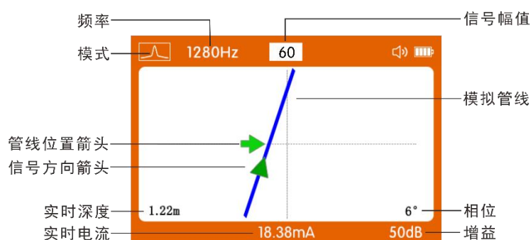
图 29 导线巡航模式界面
