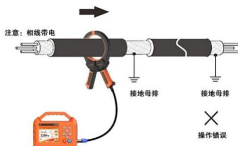
图 22 运行电缆卡钳耦合合法 1（卡电缆本体）
