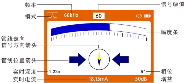
图 32 经典定位界面（2）
