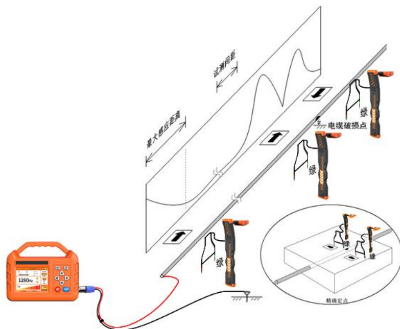
图 67 故障定位过程
