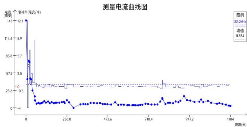
图 55 测量电流曲线图
