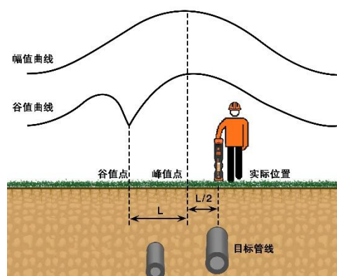
图 39 定位修正
