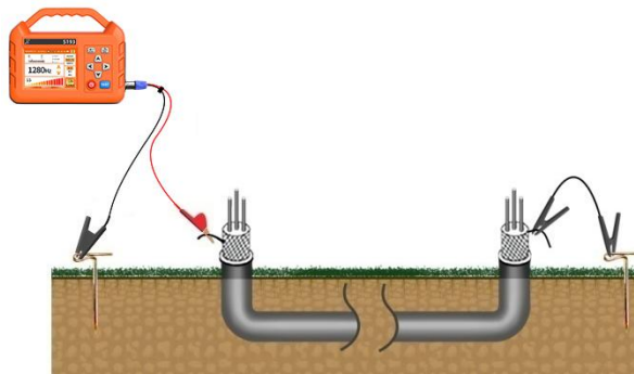
图 12 护层-大地接法接线图
