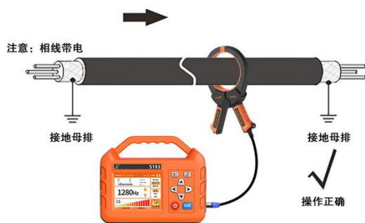
图 22 运行电缆卡钳耦合合法 1（卡电缆本体）
