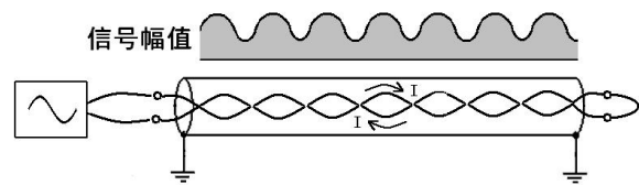
图 18 相间接法信号流向示意图
