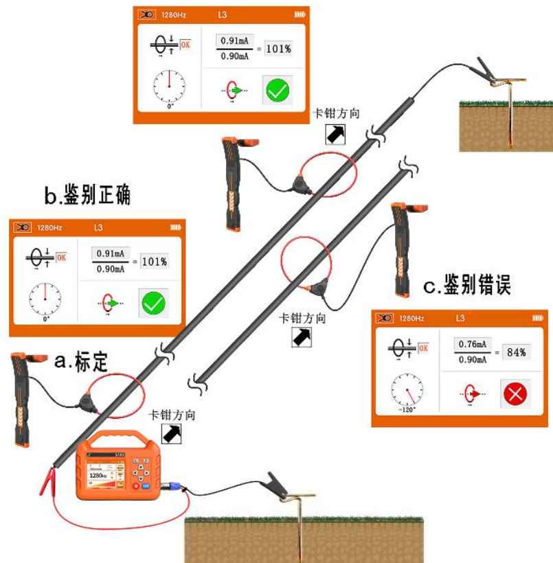
图 44 电缆识别示意图
