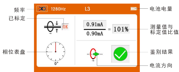
图 43 电缆识别界面
