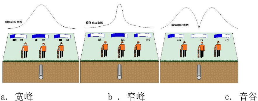
图 28 不同模式下的信号响应
