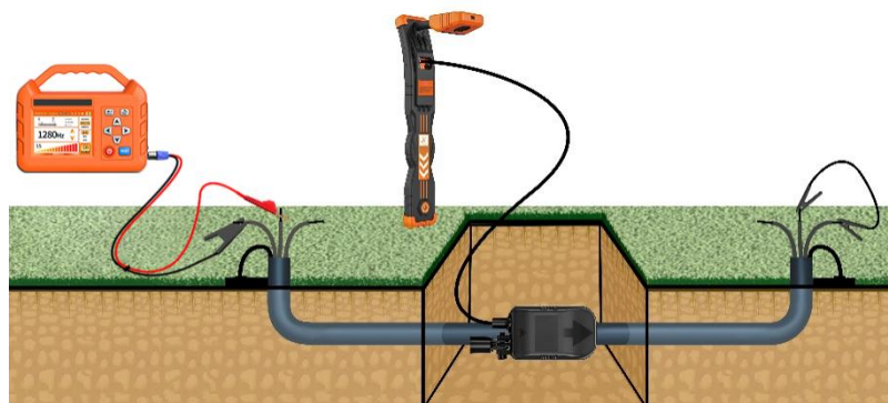
图 50 听诊器鉴别
