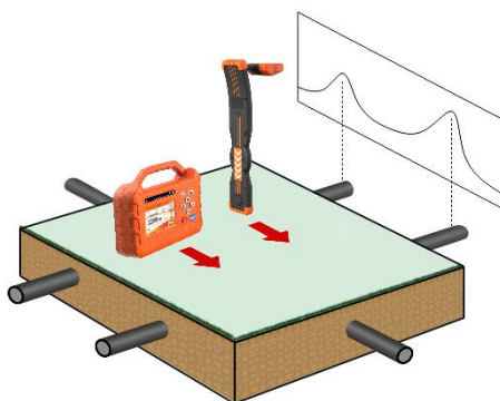
图 37 感应法区域探查
