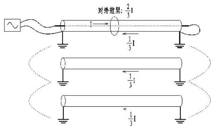
图 16 并行电缆的分流效果
