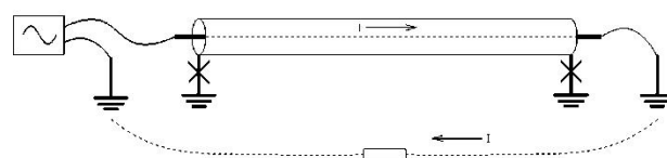
图 11 芯线-大地接法信号流向示意图
