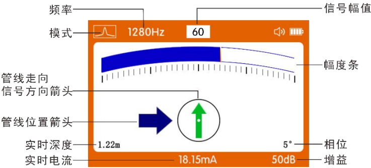
图 31 经典定位界面（1）
