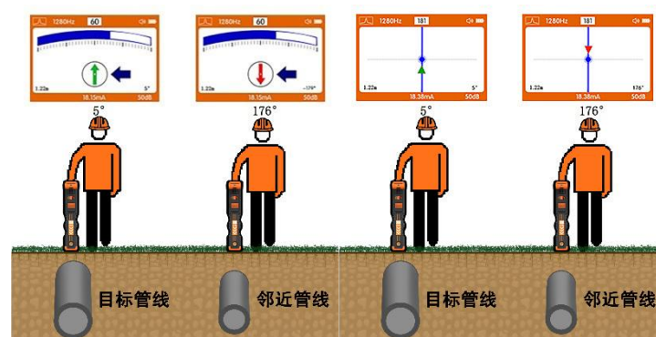
图 33 电流方向判定
