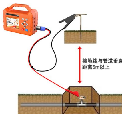
图 9 金属管道直连法接线图
