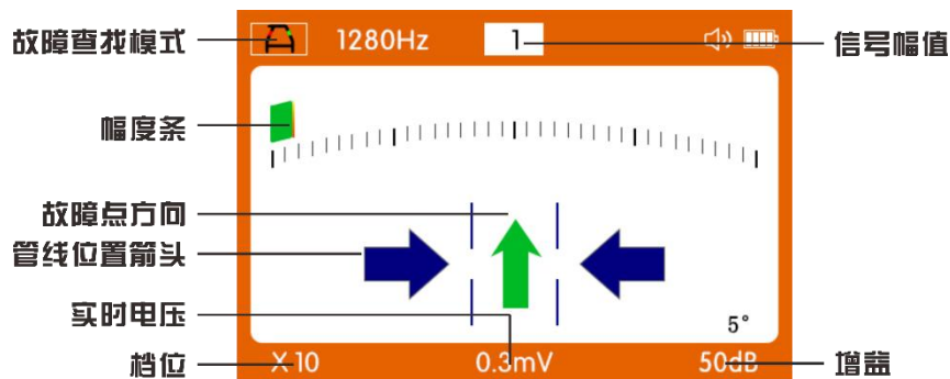
图 62 接收机故障查找界面
