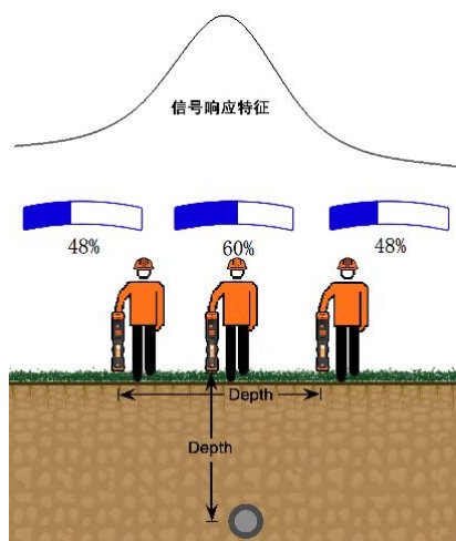
图 42 宽峰 80%法测深
