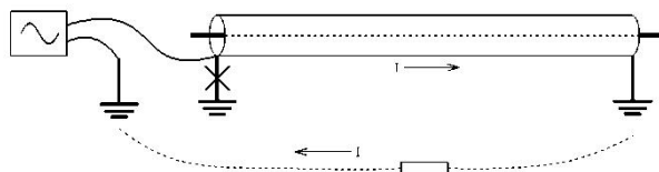
图 13 护层-大地接法信号流向示意图
